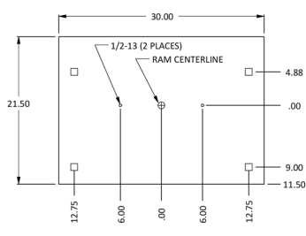
50-75 Ton
