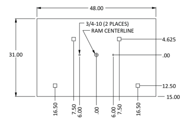
250 Ton
