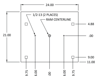
15-40 Ton
