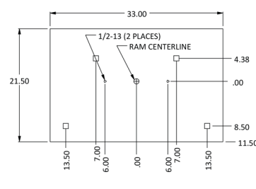
100-150 Ton
